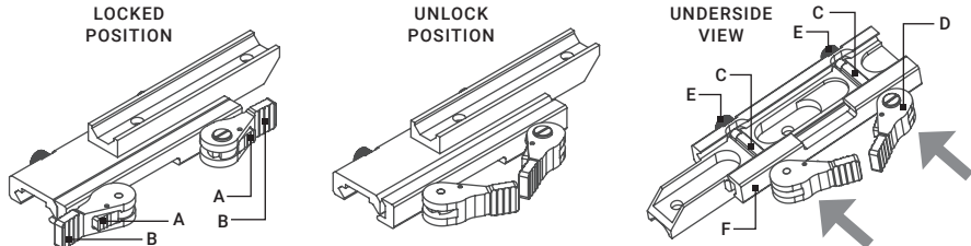
FIGURE 2-2. MOUNT.
